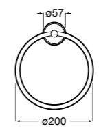
Twin 816711001 Полотенцедержатель в форме кольца. Крепление на болты или клей.
