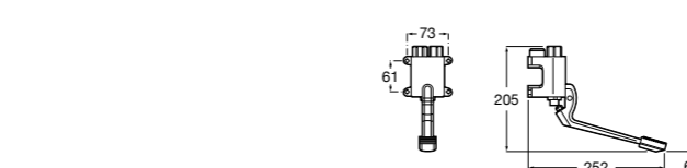
Instant Foot 505128600 Педальный смеситель. Установка на полу.
