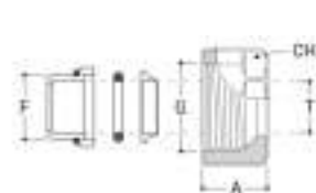
Фитинг для медной трубки
