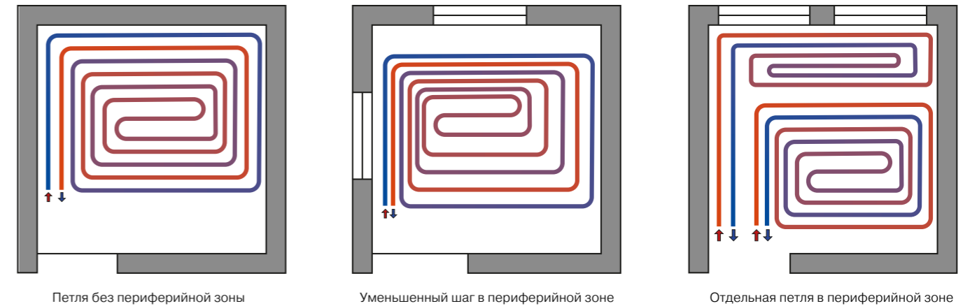
Петля без периферийной зоны Уменьшенный шаг в периферийной зоне Отдельная петля в периферийной зоне
