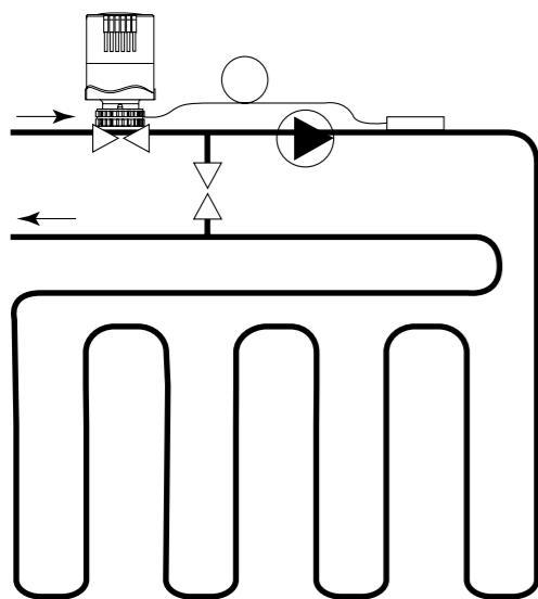
Теплый пол
