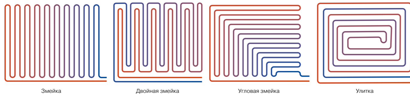
Змейка Двойная змейка Угловая змейка Улитка
