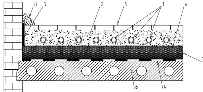
Конструкция «Мокрого тёплого пола»
