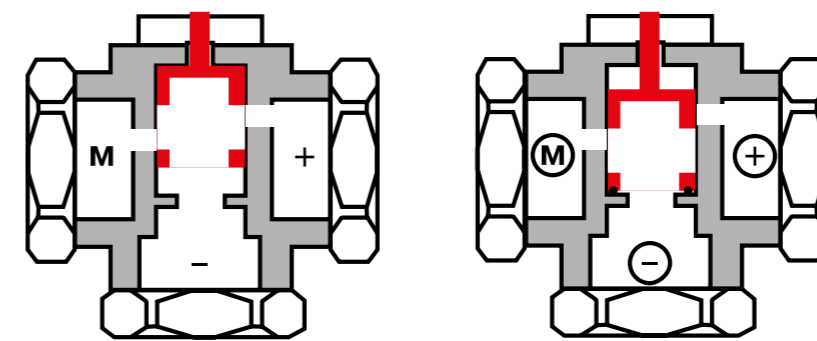
Шток в верхнем положении
