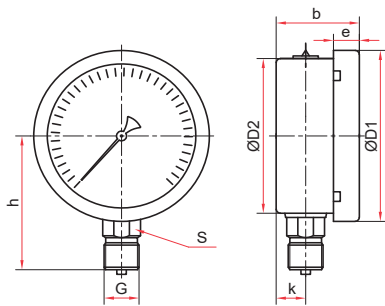
Радиальное присоединение байонетное кольцо (Ø63 мм)
