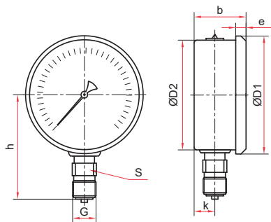
Радиальное присоединение, завальцованные (Ø40, 50, 63 мм)
