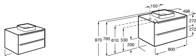
Inspira 851088XXX Мебельный модуль, совместим с полувстраиваемыми раковинами формы ROUND / SOFT. Раковина и смеситель не входят в комплект. Влагостойкая столешница. 851096XXX Мебельный модуль, совместим с полувстраиваемыми раковинами формы SQUARE. Раковина и смеситель не входят в комплект. Влагостойкая столешница. 816815339 Комплект из 2-х ножек.
