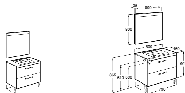
Prisma 855952XXX UNIK - Комплект мебели и раковины. Компактный сифон. Ножки и смеситель не входят в комплект. 855936XXX ПАК - Комплект мебели, раковины и зеркала Prisma Basic со встроенной LED-подсветкой. Компактный сифон. Ножки и смеситель не входят в комплект. 816764339 Комплект из 2-х ножек.
