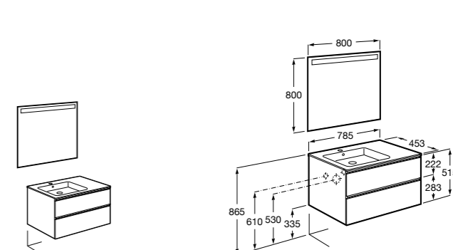
The Gap раковина слева ® 851479XXX UNIK - Комплект мебели с 2 ящиками и раковины. 851512XXX ПАК - Комплект мебели с 2 ящиками, раковины и зеркала Eidos. 816826339 Набор из 2 ножек 335 мм для мебели UNIK с 2 ящиками. 816826458 Набор из 2 ножек 335 мм для мебели UNIK с 2 ящиками.
