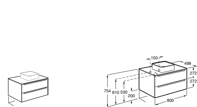
Inspira 851080XXX Мебельный модуль для накладной раковины. Раковина и смеситель не входят в комплект. Влагостойкая столешница. 816815339 Комплект из 2-х ножек.
