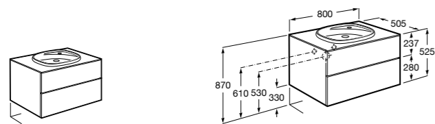
Beyond 851357XXX UNIK - Комплект мебели с двумя ящиками и раковиной из материала FINECERAMIC®. Ножки и смеситель не входят в комплект.
