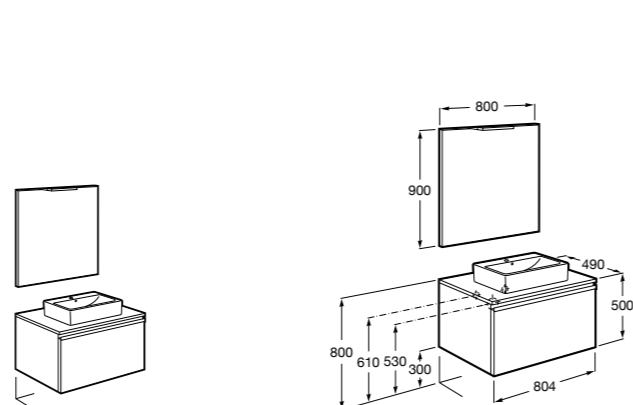
Heima 851002XXX Мебельный модуль для раковины с рабочей поверхностью. Раковина и смеситель не входят в комплект. Модуль дополнительно обработан защитой от влаги. 851040XXX ПАК - Комплект мебели, раковины и зеркала с подсветкой LED Smartlight. Компактный сифон. Раковина, ножки и смеситель не входят в комплект. Модуль дополнительно обработан защитой от влаги. 856925331 Комплект из 2-х ножек.
