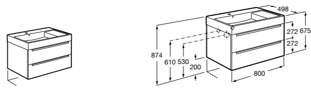
Inspira 851076XXX UNIK - Комплект мебели и раковины. Компактный сифон. Ножки и смеситель не входят в комплект. 816815339 Комплект из 2-х ножек.
