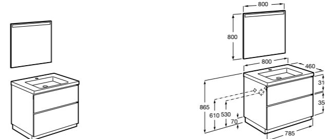
Lander 851425XXX UNIK - Комплект мебели, раковины и зеркала с подсветкой LED Smartlight. Компактный сифон. Раковина, ножки и смеситель не входят в комплект. Модуль дополнительно обработан защитой от влаги. 851430XXX ПАК - Комплект мебели, раковины и зеркала Eidos. Ножки и смеситель не входят в комплект. Встроенная розетка. Модуль дополнительно обработан защитой от влаги. 816824339 Комплект из 2-х ножек.
