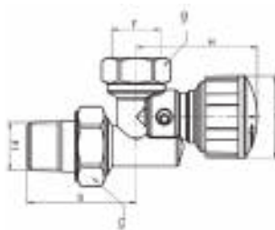
Клапан термостатический осевой
