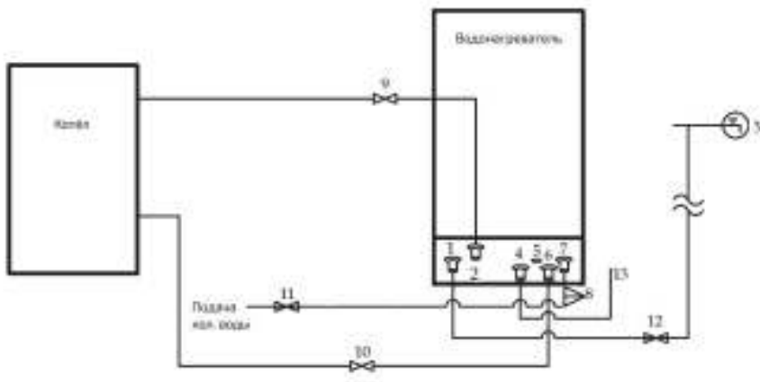
Рисунок 2. Подключение КЭВН
