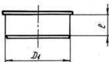
Рисунок 9 - Заглушка
