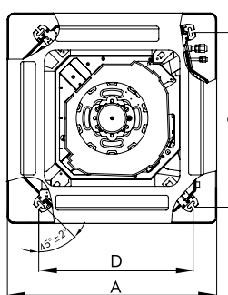
Внешние размеры панели
