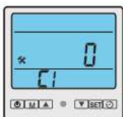
Параметры C1 Значение кода: Текущая погода с функцией обогрева 0: НЕТ 1: ДА Согласие: 0
