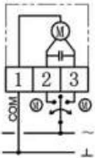
Электрическая схема ARV-1000VR
