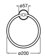
Twin 816711001 Полотенцедержатель в форме кольца. Крепление на болты или клей.
