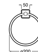
Victoria 816659001 Полотенцедержатель в форме кольца. Крепление на болты или клей.
