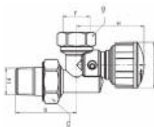
Клапан термостатический осевой
