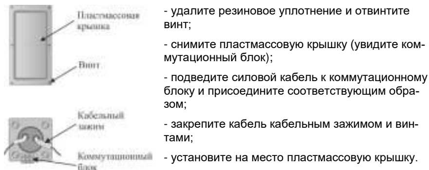
Рисунок 2. Подключение к блоку коммутации.
