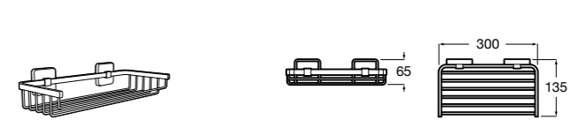
Victoria 816688001 Контейнер решетчатый. Крепление на болты или клей.
