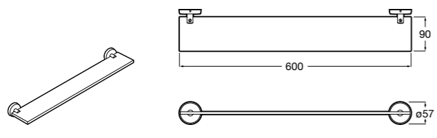
Twin 816708001 Полочка. Крепления в комплекте.
