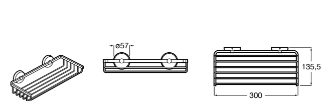
Twin 816714001 Контейнер. Крепление на болты или клей.
