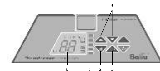
Рис. 2 Панель управления
