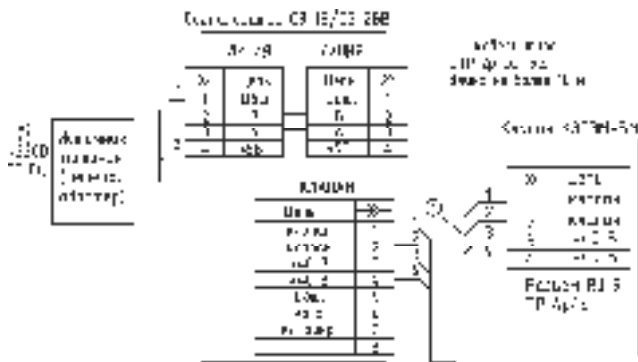
Рис. А2. Схема электрических соединений сигнализаторов СЗ-Б и бытового электромагнитного клапана КЗГЭМ-Б(без узла индикации положения клапана).
