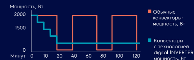
РИС.1 АВТОМАТИЧЕСКОЕ ИЗМЕНЕНИЕ МОЩНОСТИ ДЛЯ ЭКОНОМИИ ЭЛЕКТРОЭНЕРГИИ
