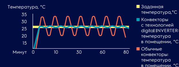
РИС.2 ТОЧНОСТЬ ПОДДЕРЖАНИЯ ТЕМПЕРАТУРЫ
